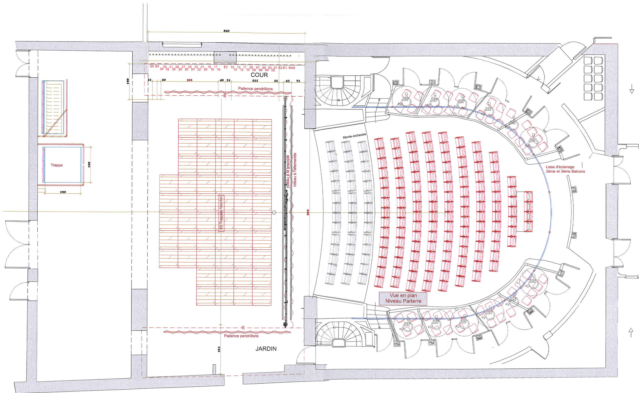
THEATRE DE LA COUPE D'OR - ROCHEFORT DOE Equipements Machinerie scénique Plan du Parterre - ech 1/100e - le 01/10/12
