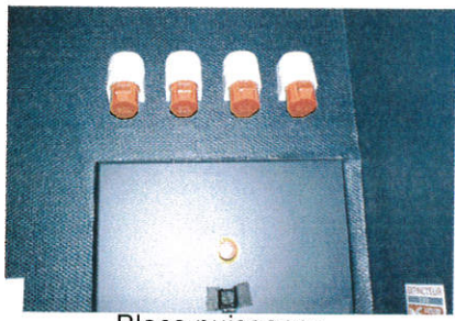
Blocs puissance
