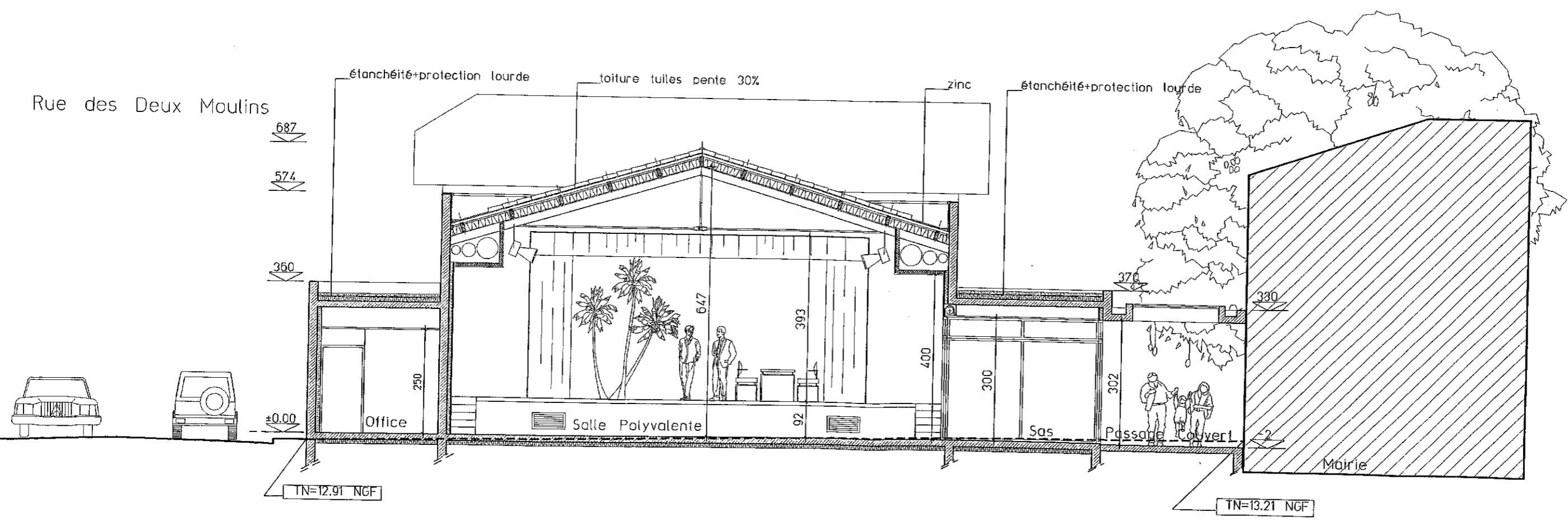
Coupe sur Salle Polyvalente
